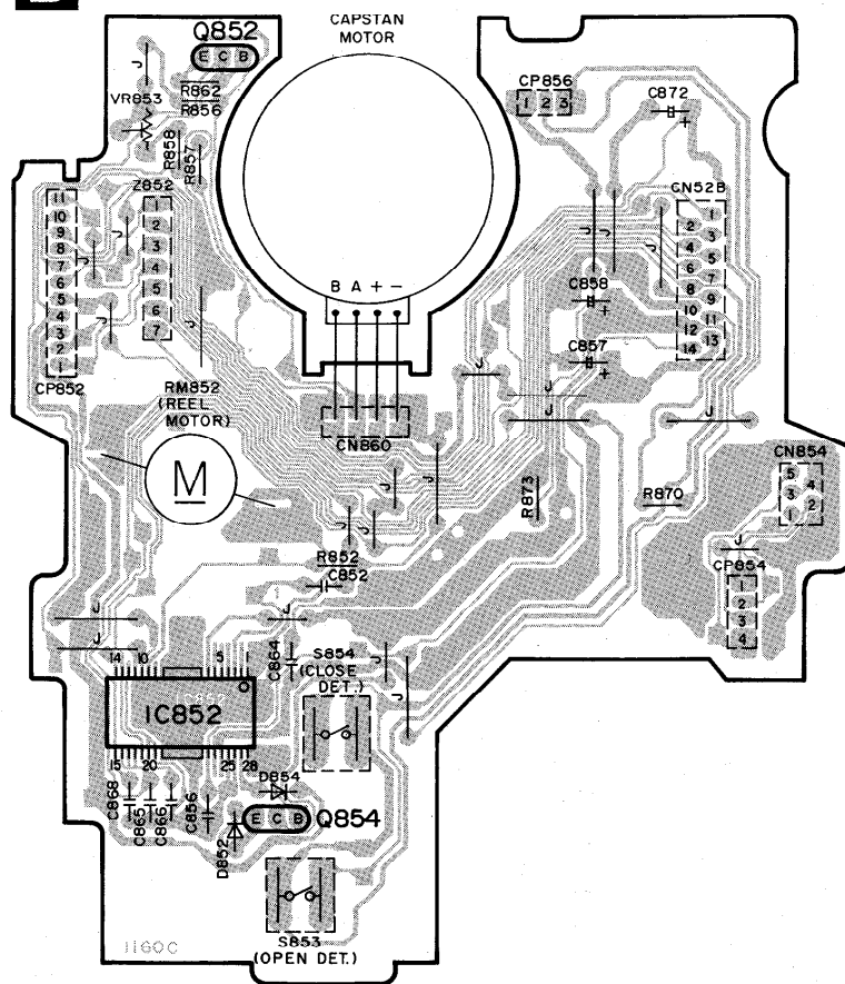
B モーター基板 (DECK1)
