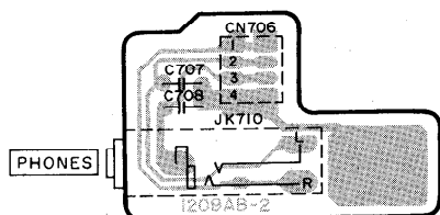
H ヘッドホン ジャック基板
