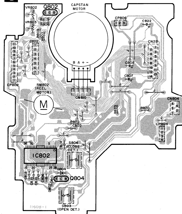
C モーター基板 (DECK2)
