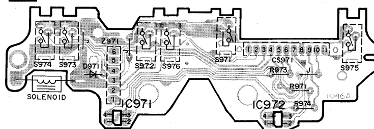
E メカニズム基板 (DECK1)
